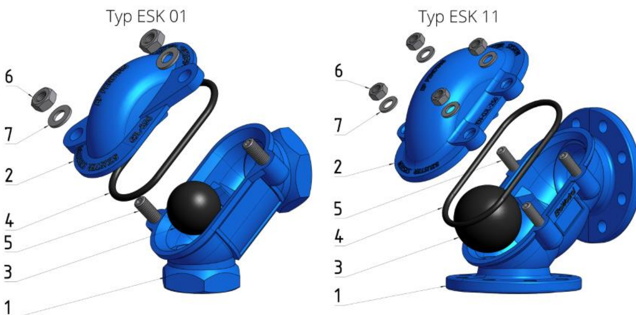
Rys.1 Wykaz części zamiennych zaworów ESK 01 i ESK 11
